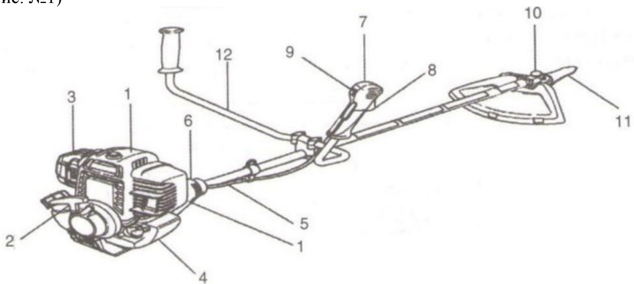
Рис. 1. Ручная газонокосилка:
